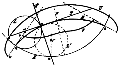
Č. 1881. Hypocykloida.
